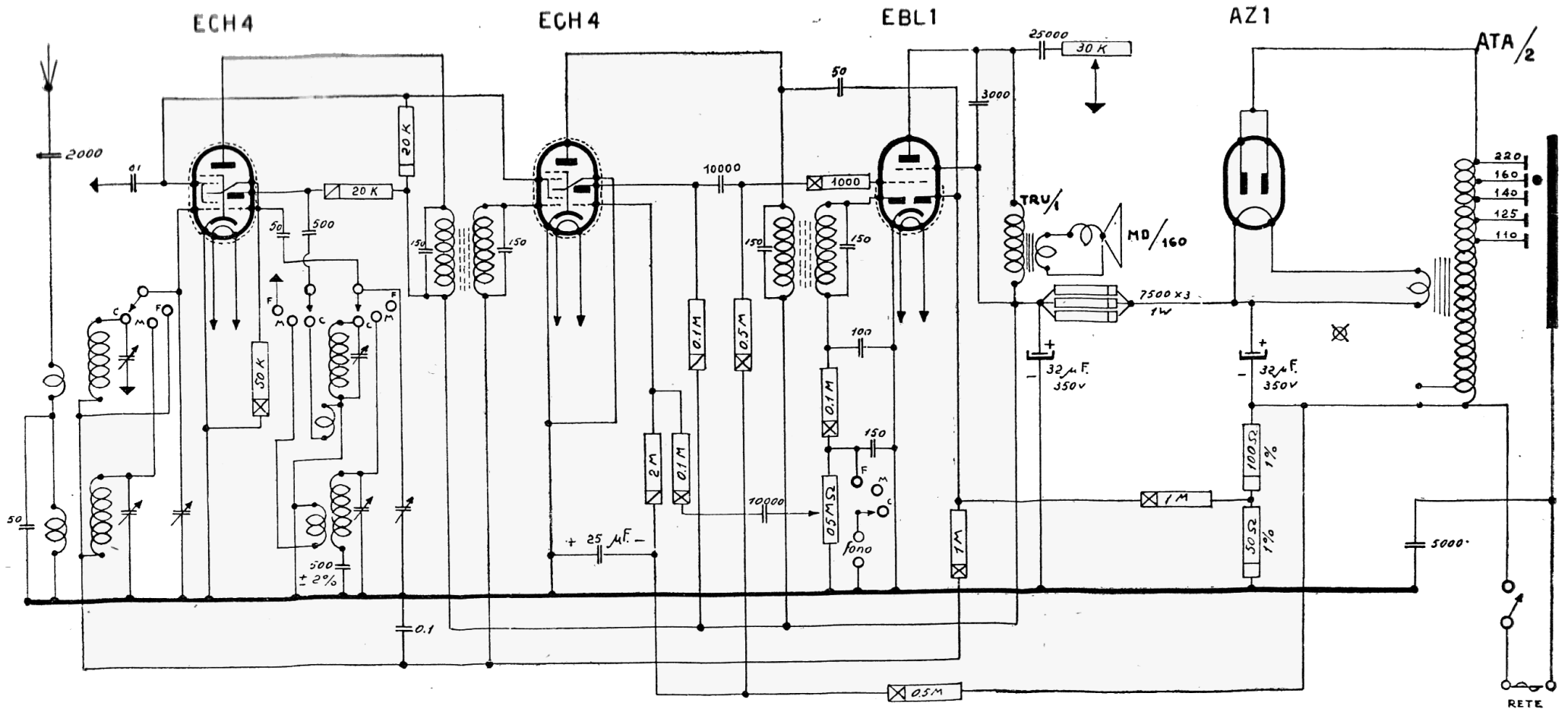
BERTONCINI RADIO - Mod. TOTI 1, mod. TOTI 2 e mod. TOTI 52. Onde medie e corte. Il triodo della seconda ECH4 provvede all'amplificazione di tensione BF. Media frequenza: 468 kc. Altoparlante a magnete permanente. Un capo della rete-luce è collegato al telaio.
